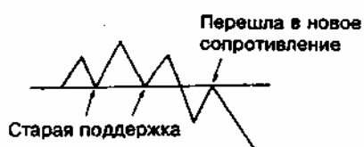
Рис. 11.22. Изменение полярности: поддержка переходит в сопротивление
